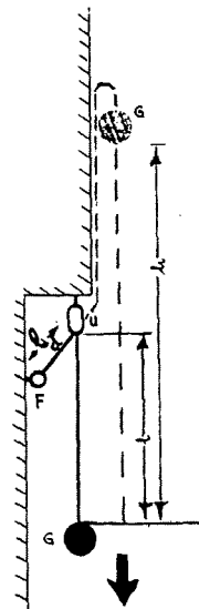
Schema der UIAA-Sturzprüfung
